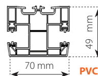
Geleider dubbel - Coulisse double
